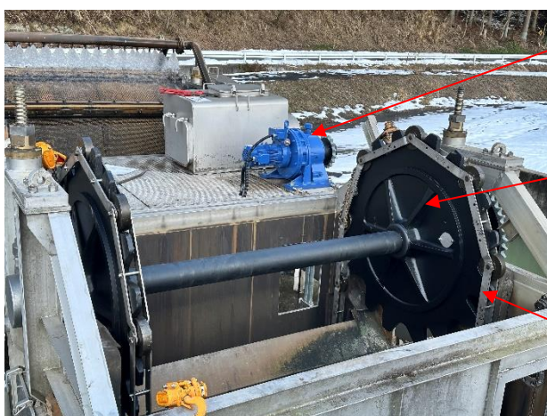
▲キャリングチェーン・ホイール等の更新
